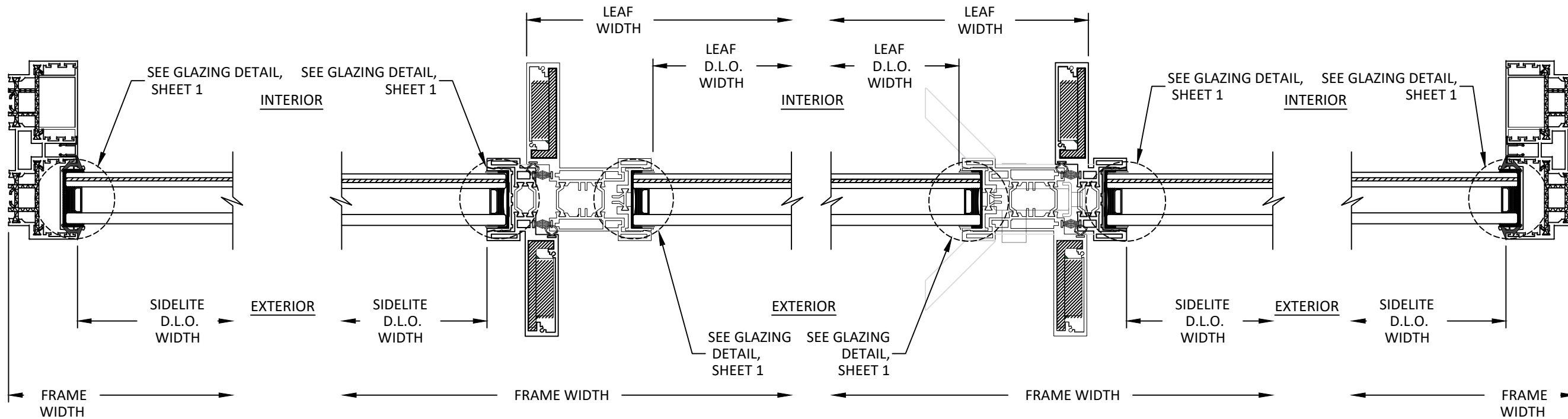
D 8 HORIZONTAL SECTION SIDELITE JAMB
